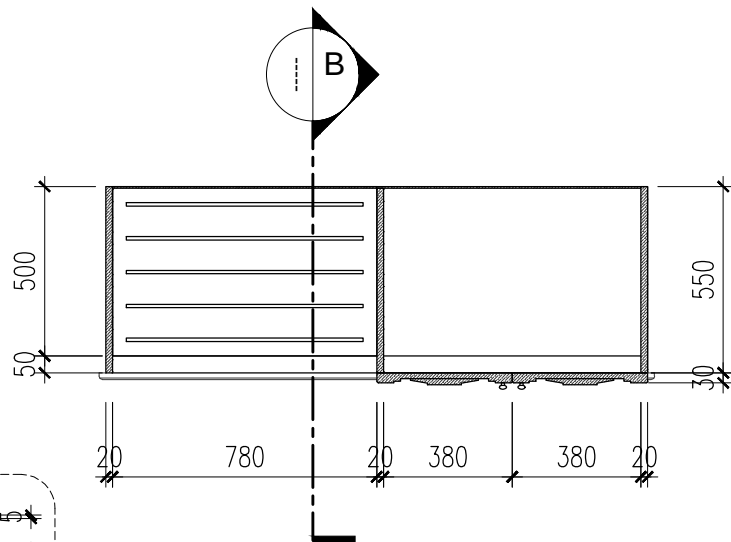
B MẶT CẮT A TỶ LỆ 1:50
