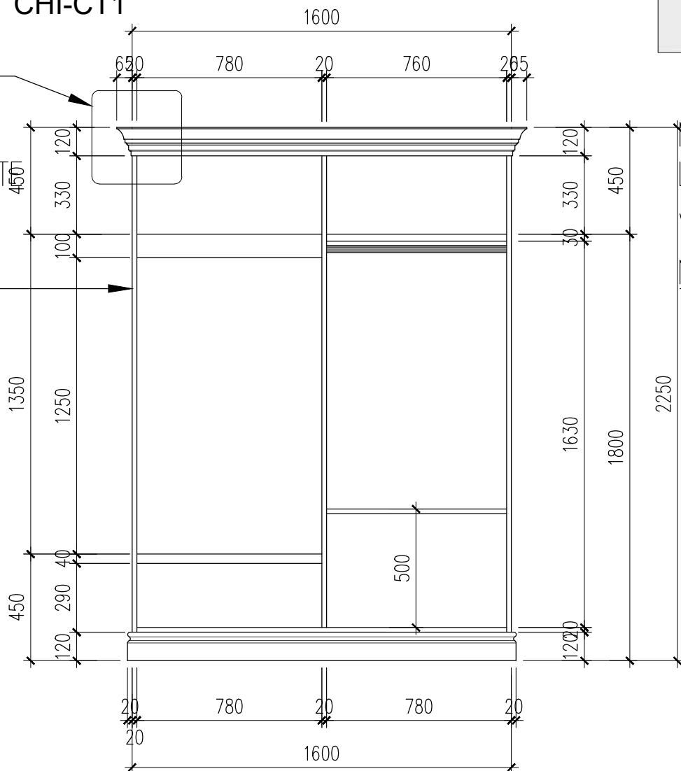
D MẶT ĐỨNG TRONG TỶ LỆ 1:50
