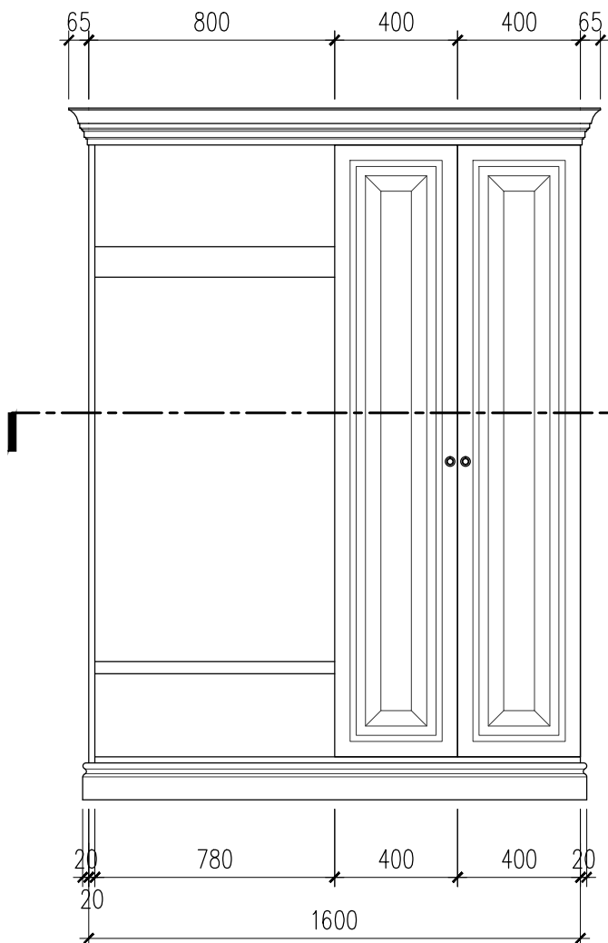
C MẶT ĐỨNG TRƯỚC TỶ LỆ 1:50
