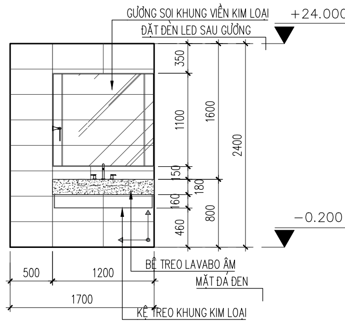
B MẶT ĐỨNG A TỶ LỆ 1/100
