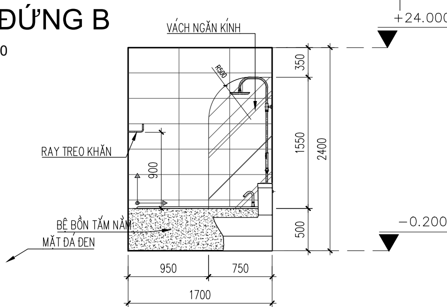
D MẶT ĐỨNG C TỶ LỆ 1/100
