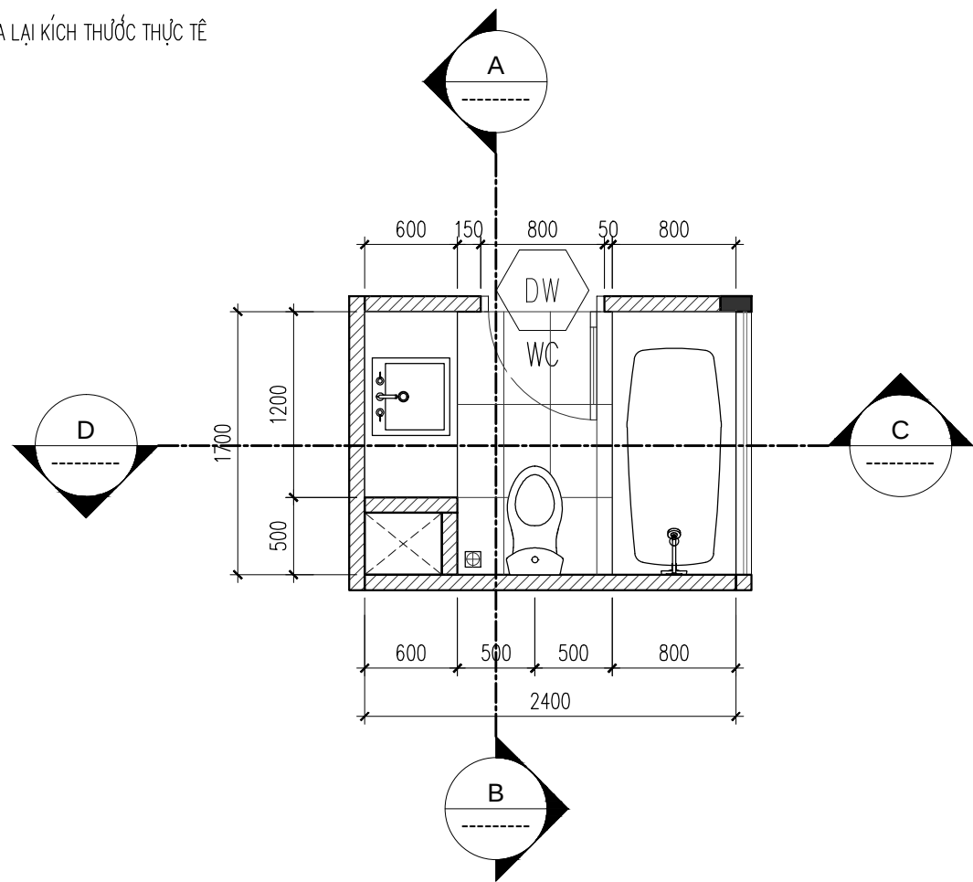
A MẶT BẰNG TỶ LỆ 1/100
