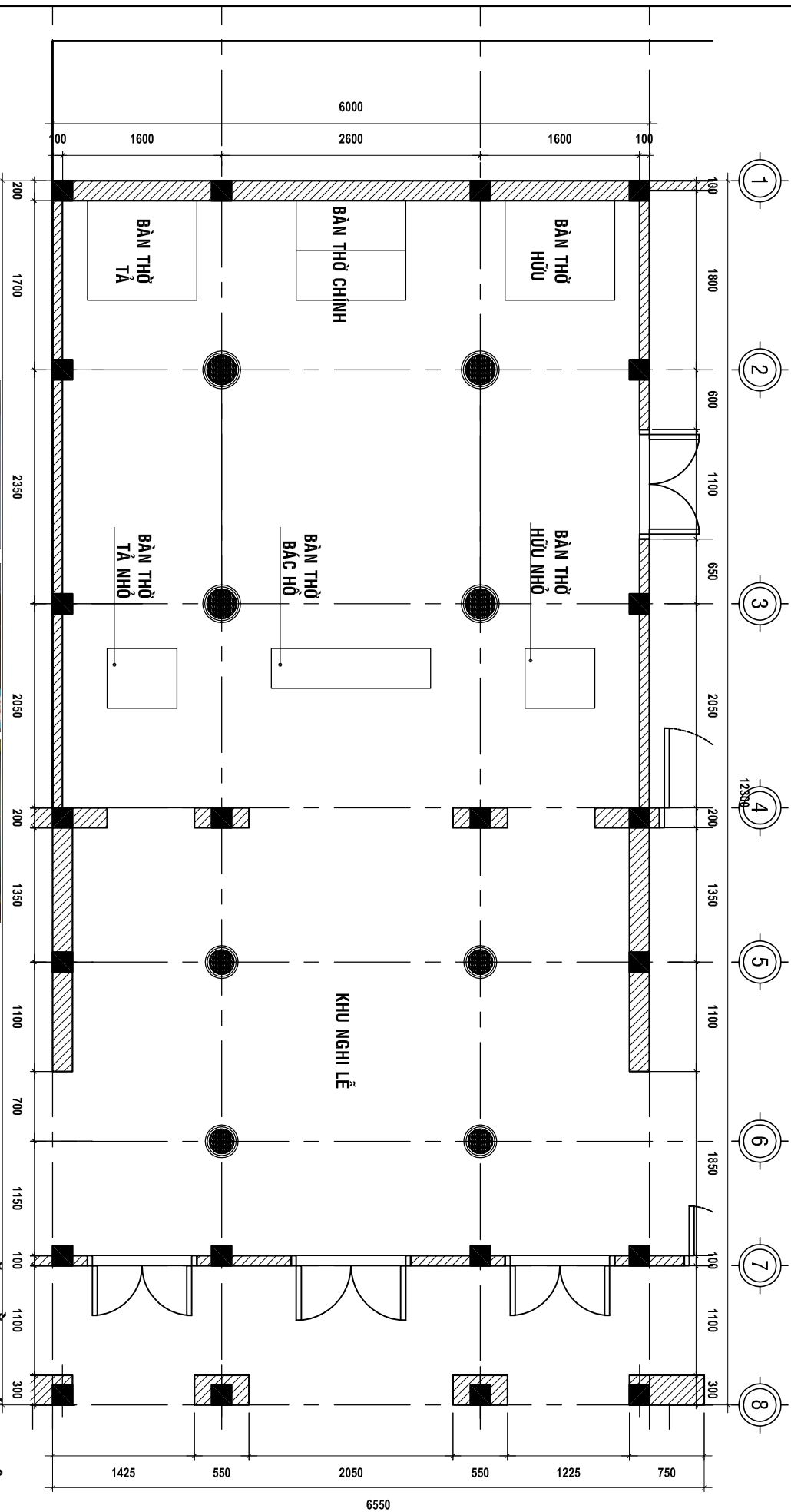
MẶT BẰNG CHÍNH ĐIỆN TỈ LỆ : 1/ 80
