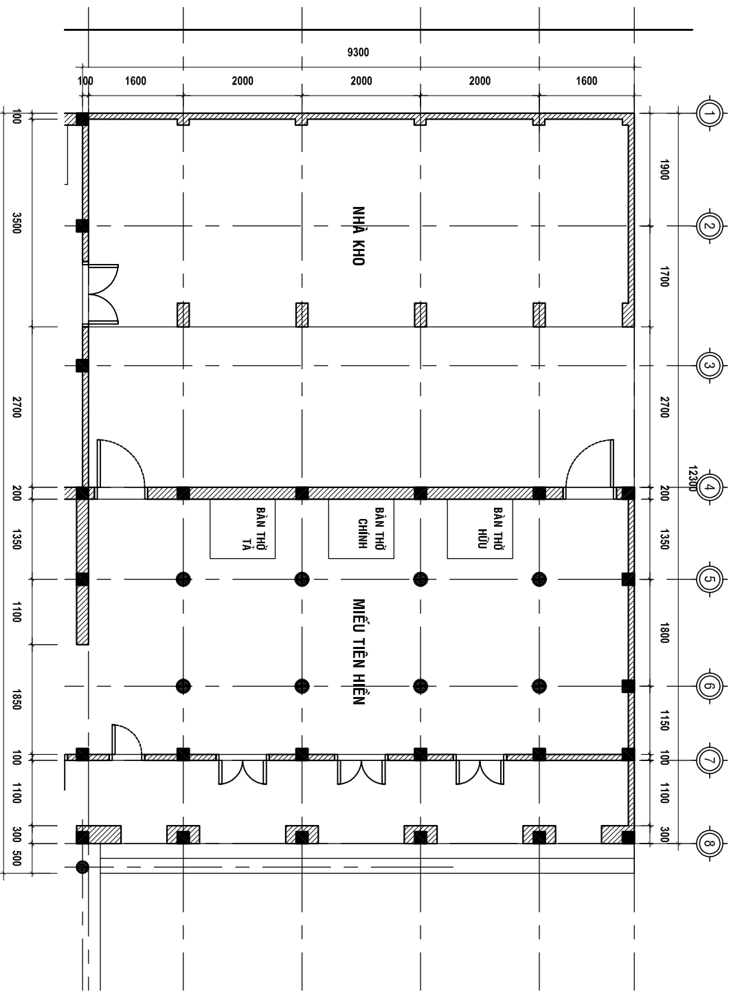
MẶT BẰNG MIẾU TIỀN HIỂN TỈ LỆ : 1/ 120
